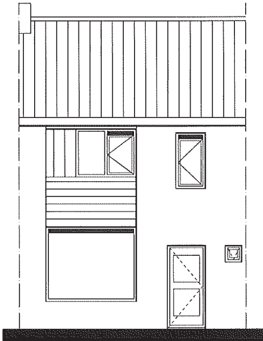
VOORGEVEL
