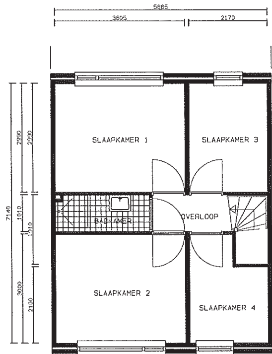
EERSTE VERDIEPING
