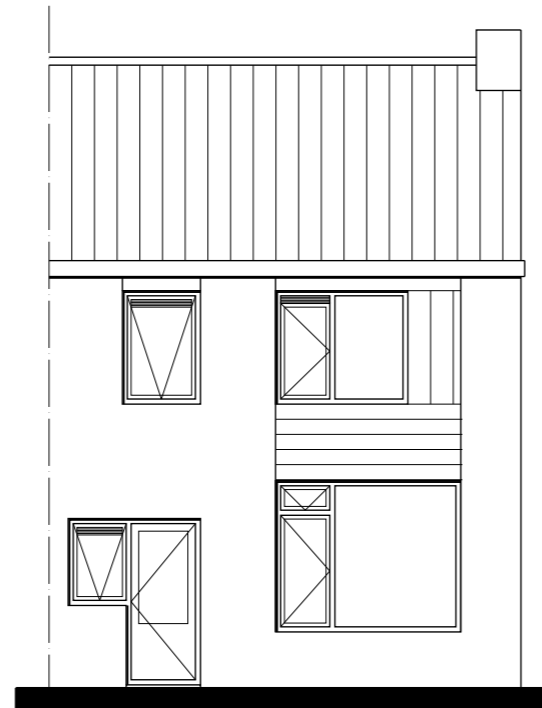
ACHTERGEVEL
