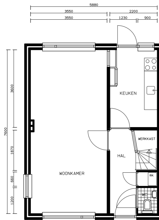
BEGANE GROND
