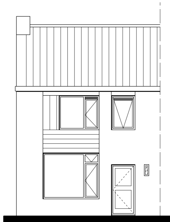
VOORGEVEL
